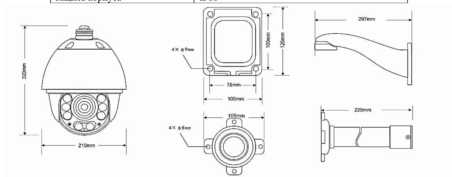
Рисунок А.36 – Габаритный чертеж видеокамеры ИВМ-711.
