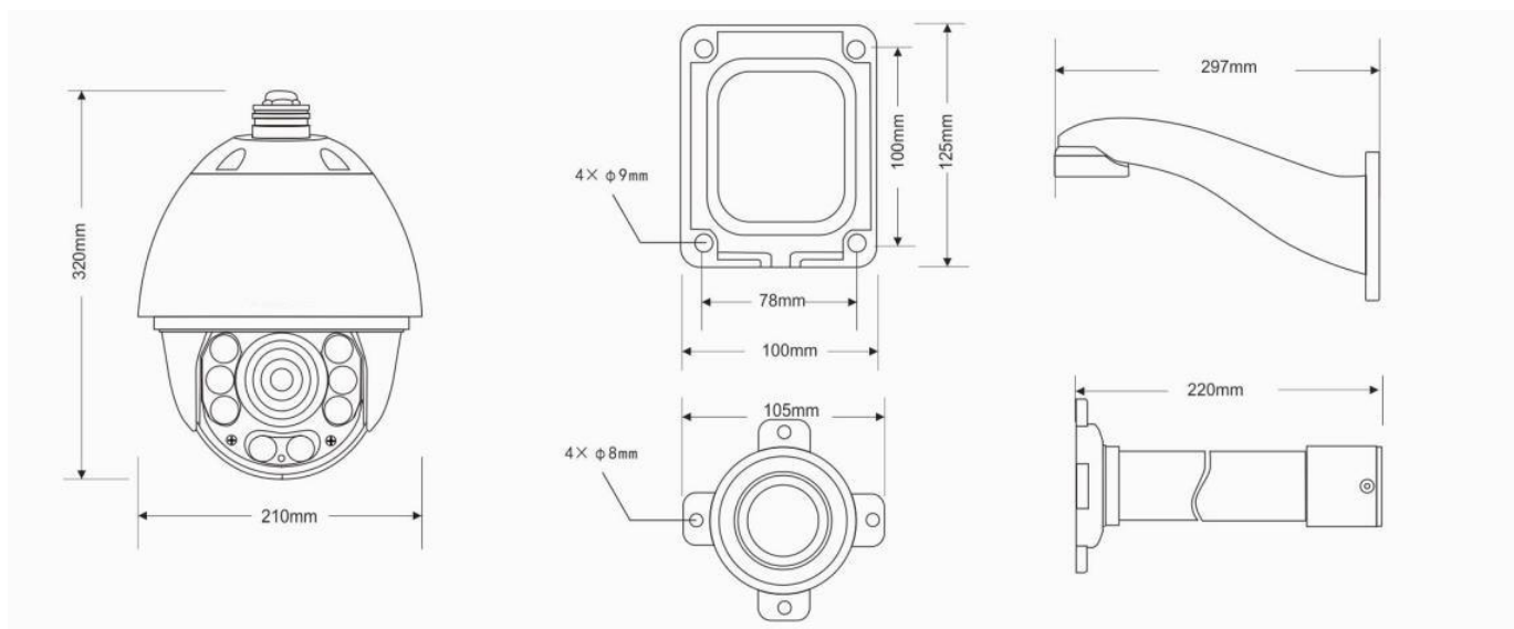
Рисунок А.44 – Габаритный чертеж видеокамеры ИВМС-601.
