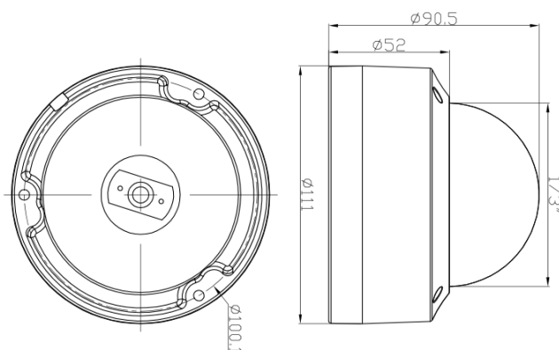
Рисунок А.26 – Габаритный чертеж видеокамеры ИВМ-401.
