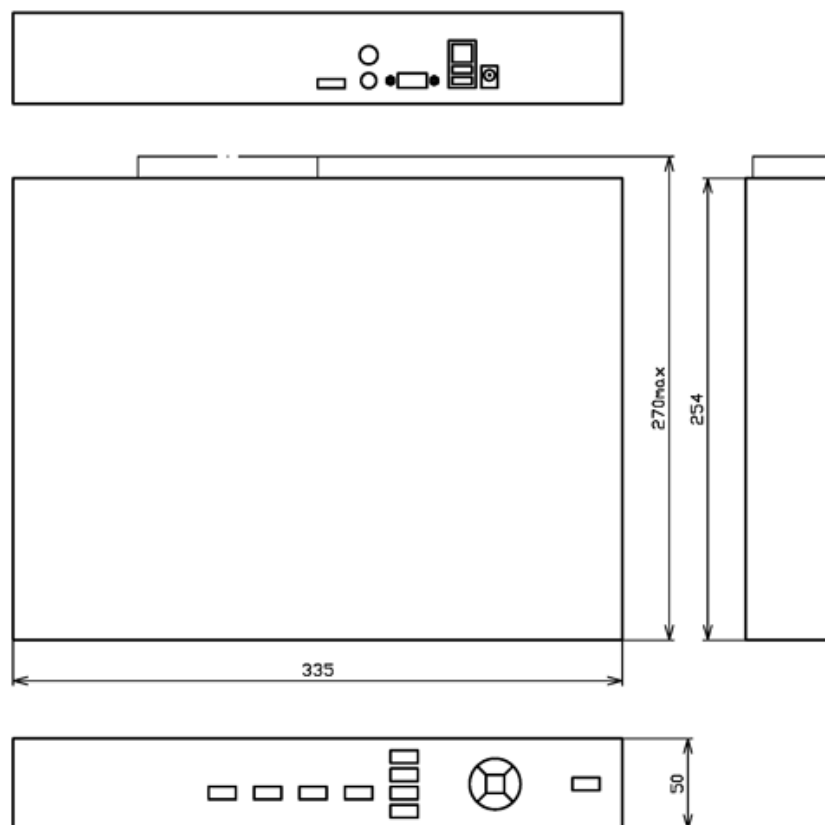
Рисунок А.24 – Габаритный чертеж видеорегистраторов ИВМС-8016, ИВМС-8032.
