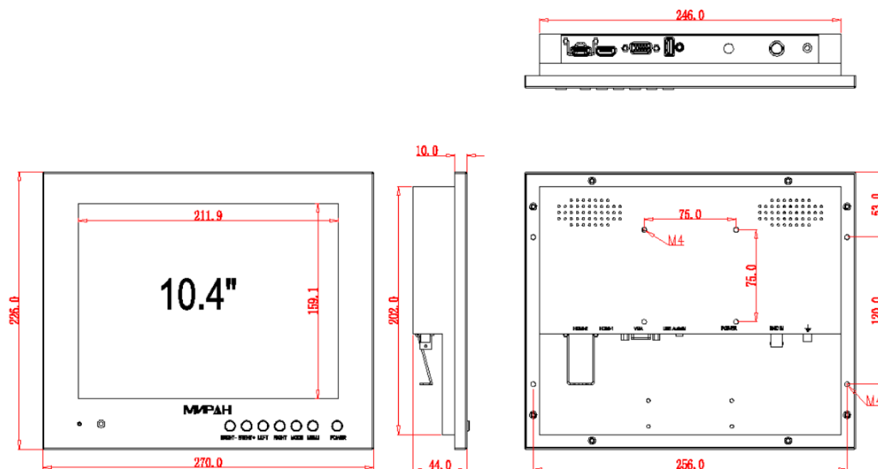
Рисунок А.50 – Габаритный чертеж монитора ИВМ-10ЖК.
