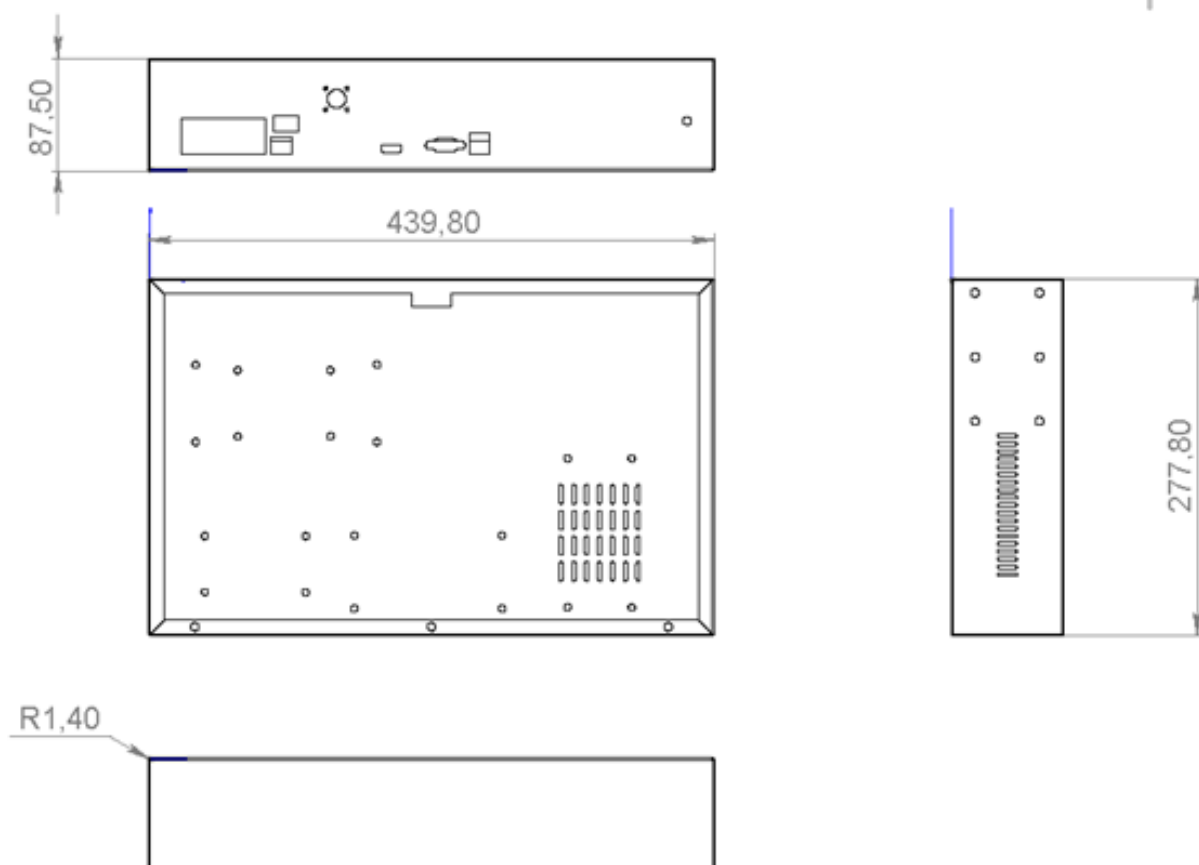
Рисунок А.15 – Габаритный чертеж видеорегистратора ИВМС-8004.
