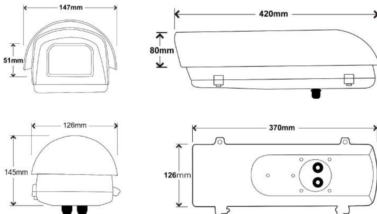
Рисунок А.34 – Габаритный чертеж видеокамеры ИВМ-602.
