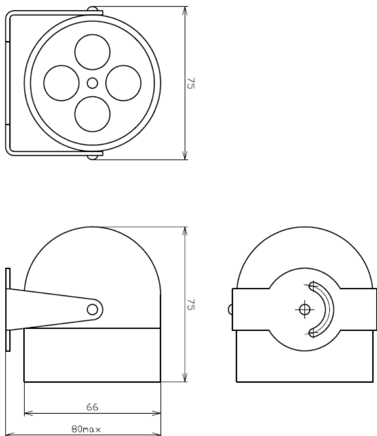
Рисунок А.62 – Габаритный чертеж прожектора ИК-601-40.
