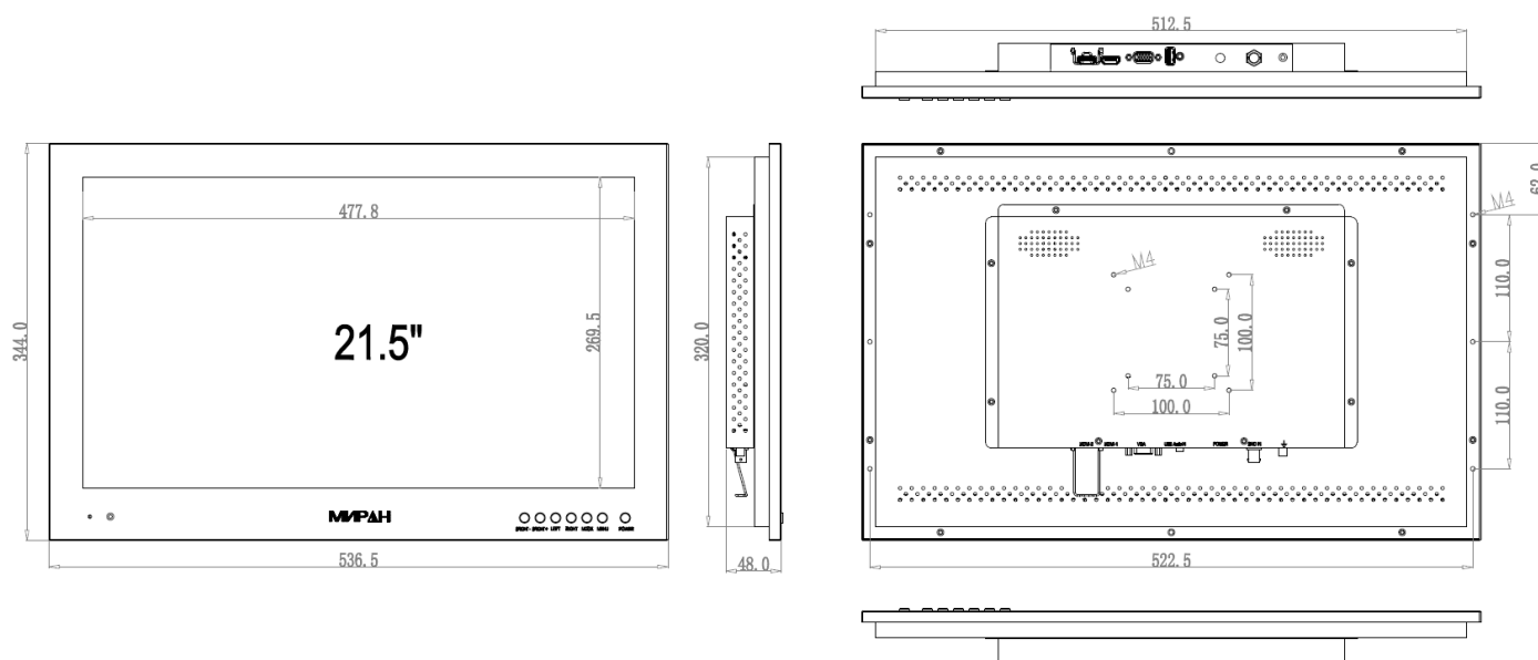
Рисунок А.60 – Габаритный чертеж монитора ИВМ-22ЖК.
