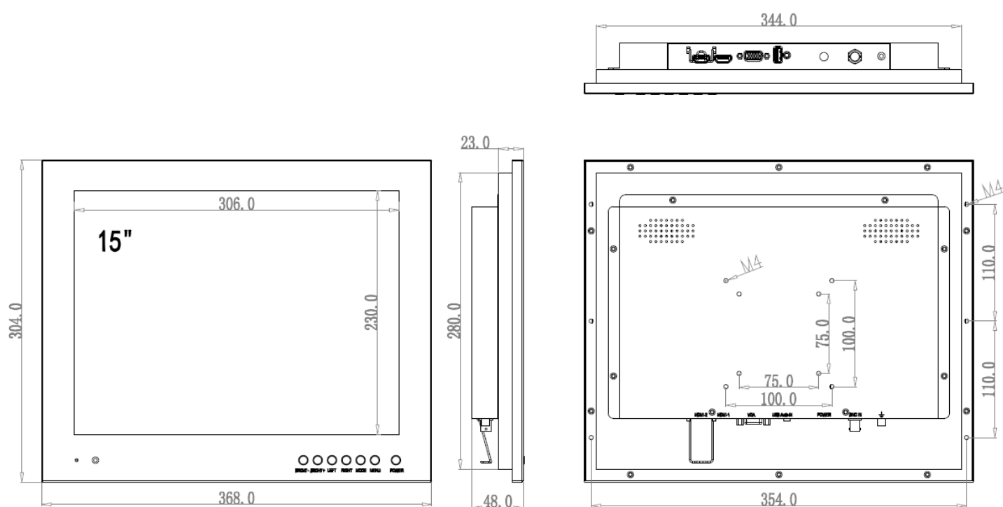
Рисунок А.54 – Габаритный чертеж монитора ИВМ-15ЖК.
