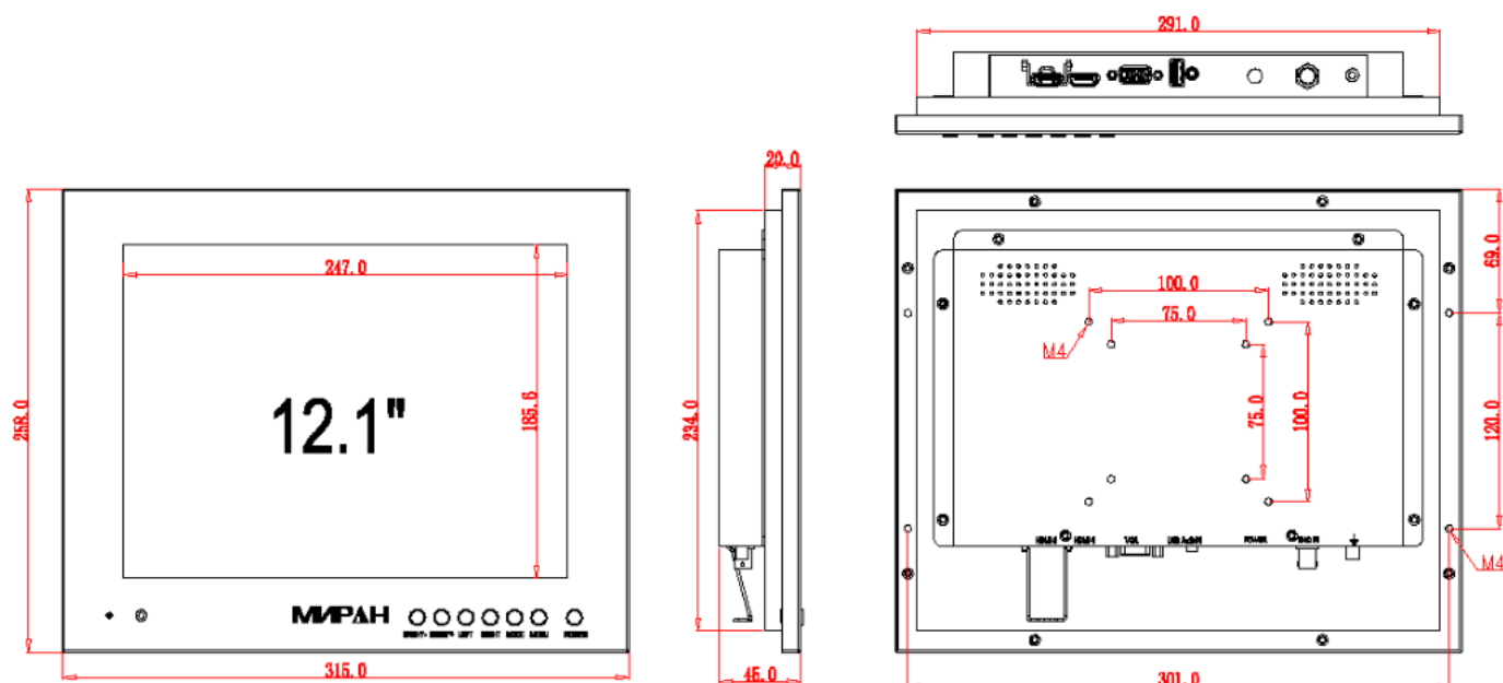
Рисунок А.52 – Габаритный чертеж монитора ИВМ-12ЖК.
