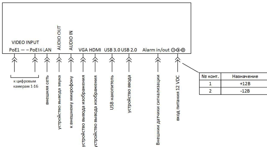
Рисунок А.20 – Схема подключения видеорегистраторов ИВМС-8016
