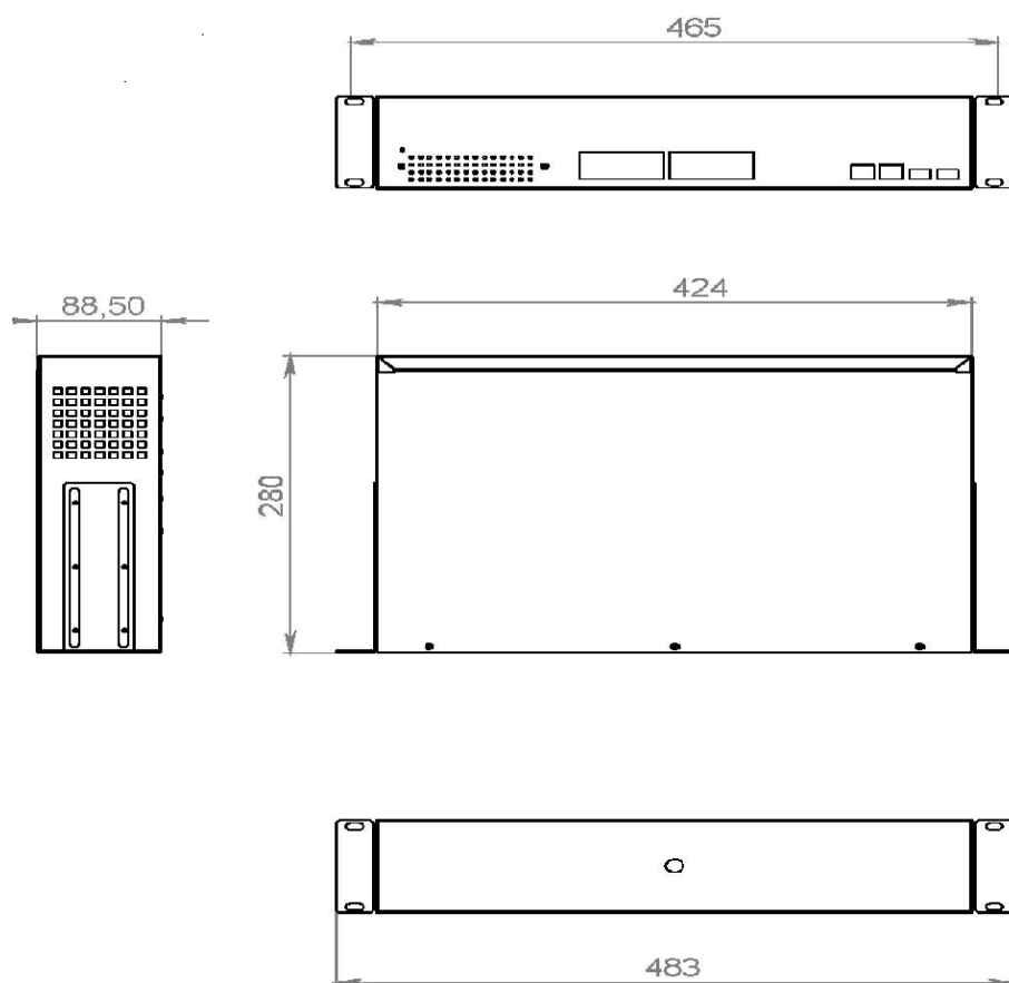
Рисунок А.48 – Габаритный чертеж коммутатора ИВК-16.
