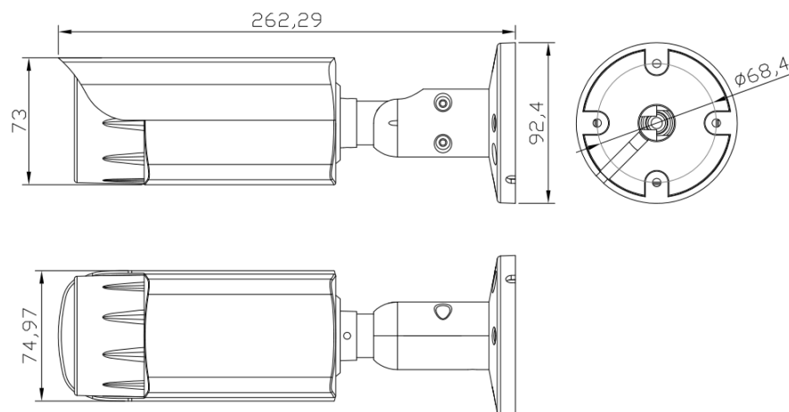
Рисунок А.28 – Габаритный чертеж видеокамеры ИВМ-501.
