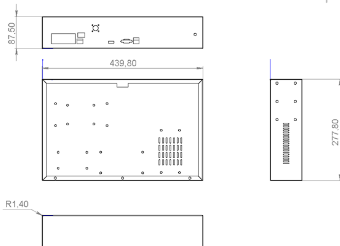
Рисунок А.21 – Габаритный чертеж видеорегистратора ИВМС-8016.
