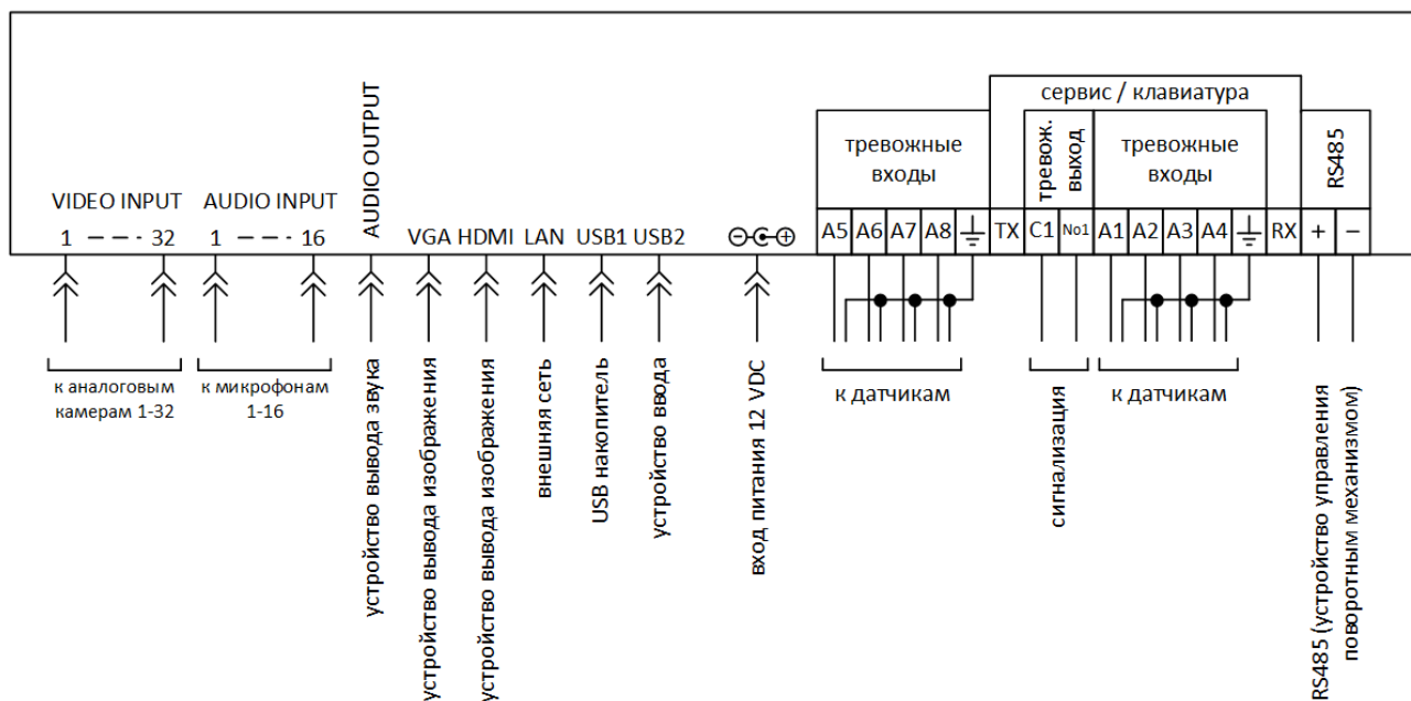
Рисунок А.11 – Схема подключения видеорегистратора ИВМ-8032.
