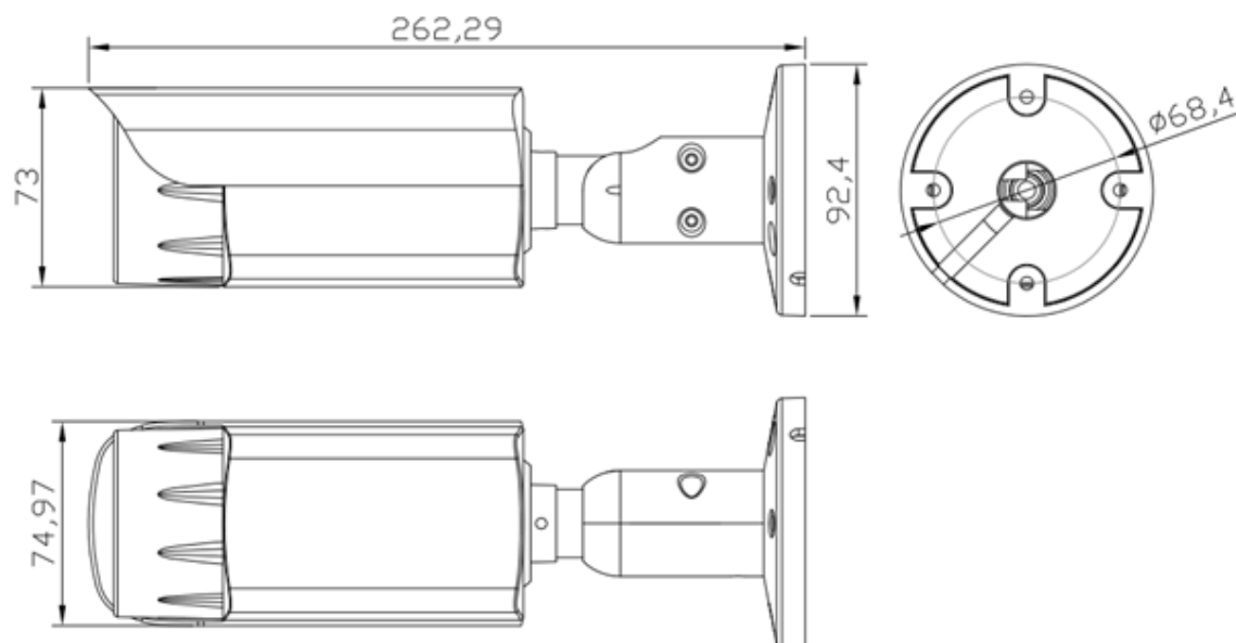
Рисунок А.40 – Габаритный чертеж видеокамеры ИВМС-501.
