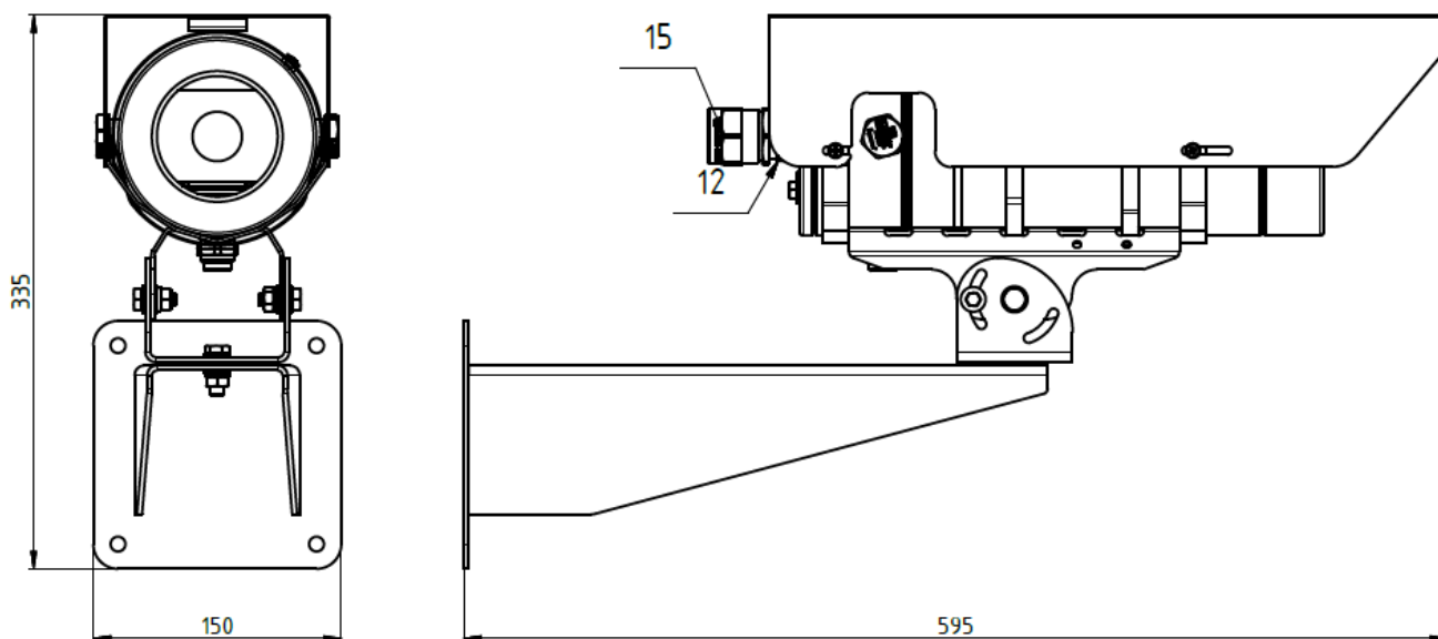
Рисунок А.32 – Габаритный чертеж видеокамеры ИВМ-501В.
