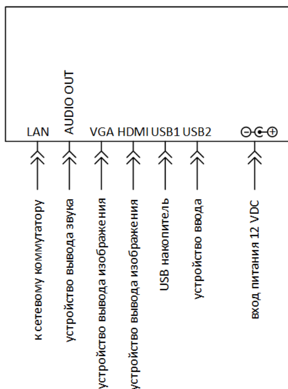
Рисунок А.23 – Схема подключения видеорегистраторов ИВМС-8016, ИВМС-8032.
