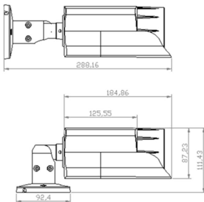
Рисунок А.30 – Габаритный чертеж видеокамеры ИВМ-501М.
