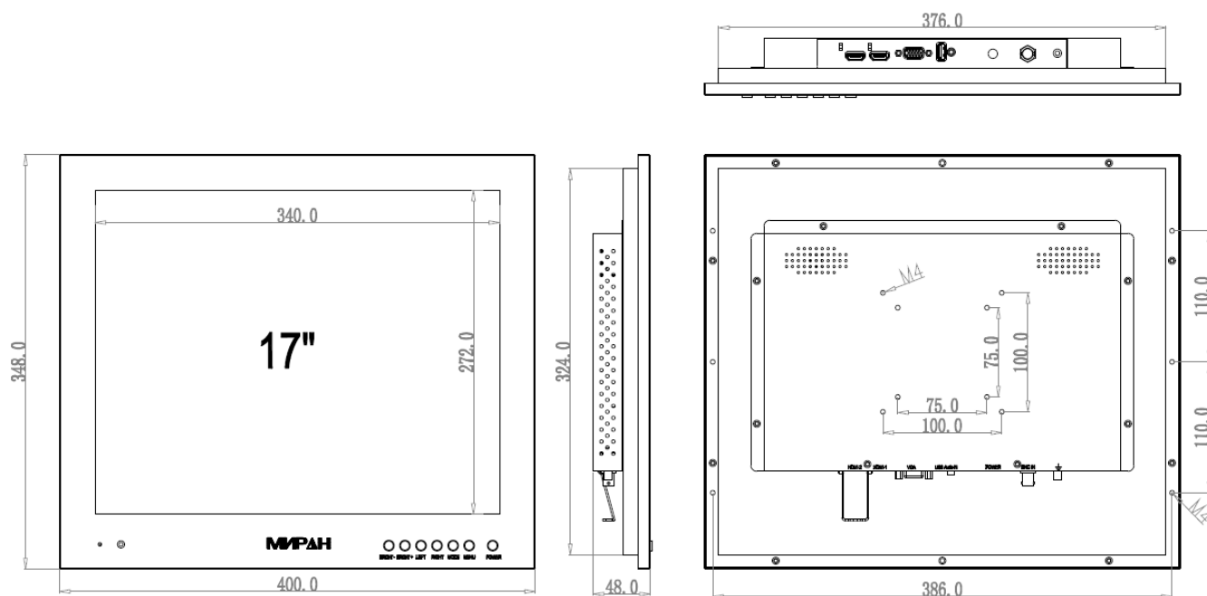
Рисунок А.56 – Габаритный чертеж монитора ИВМ-17ЖК.
