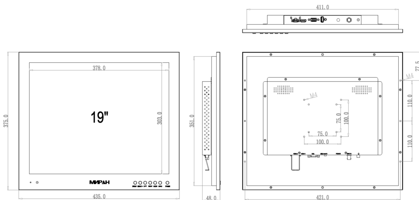
Рисунок А.58 – Габаритный чертеж монитора ИВМ-19ЖК.
