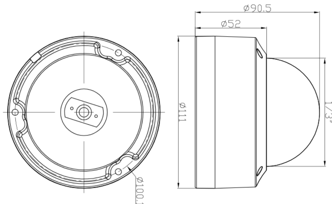
Рисунок А.38 – Габаритный чертеж видеокамеры ИВМС-401.
