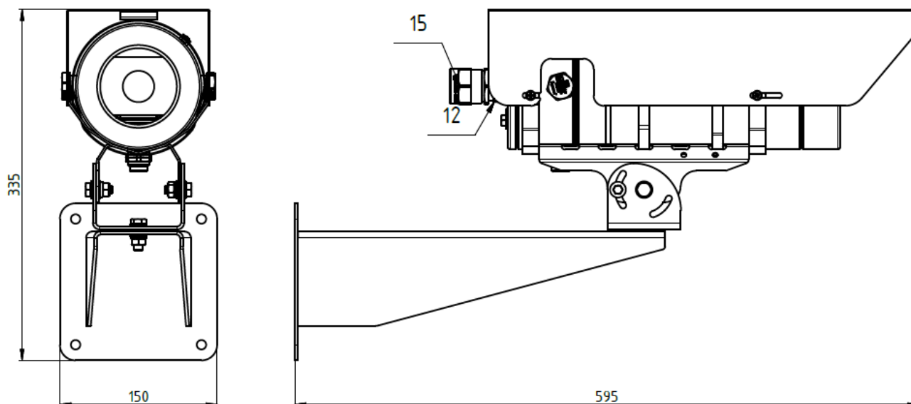
Рисунок А.42 – Габаритный чертеж видеокамеры ИВМС-501В.
